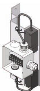
contact début et fin de course pour Hpa > 828mm position : bas de l'ouvrant REF.: O40566
