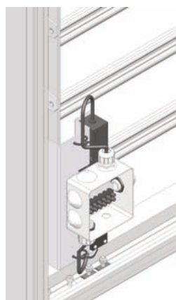
contact début et fin de course pour Hpa > 828mm position : bas de l'ouvrant REF.: O40566
