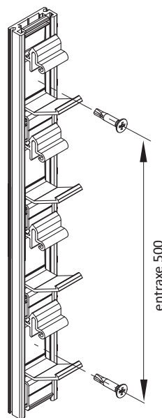
fixation direct sur le support par vis autoperceuse diam 4.8 maxi (non fournie)
