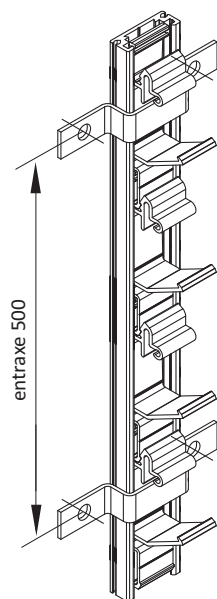
fixation par oméga en acier galvanisé
