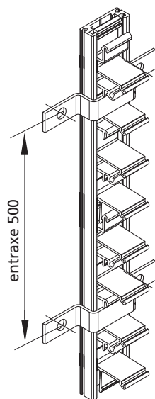
fixation par oméga en acier galvanisé
