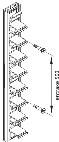
fixation direct sur le support par vis autoperceuse diam 4.8 maxi (non fournie)
